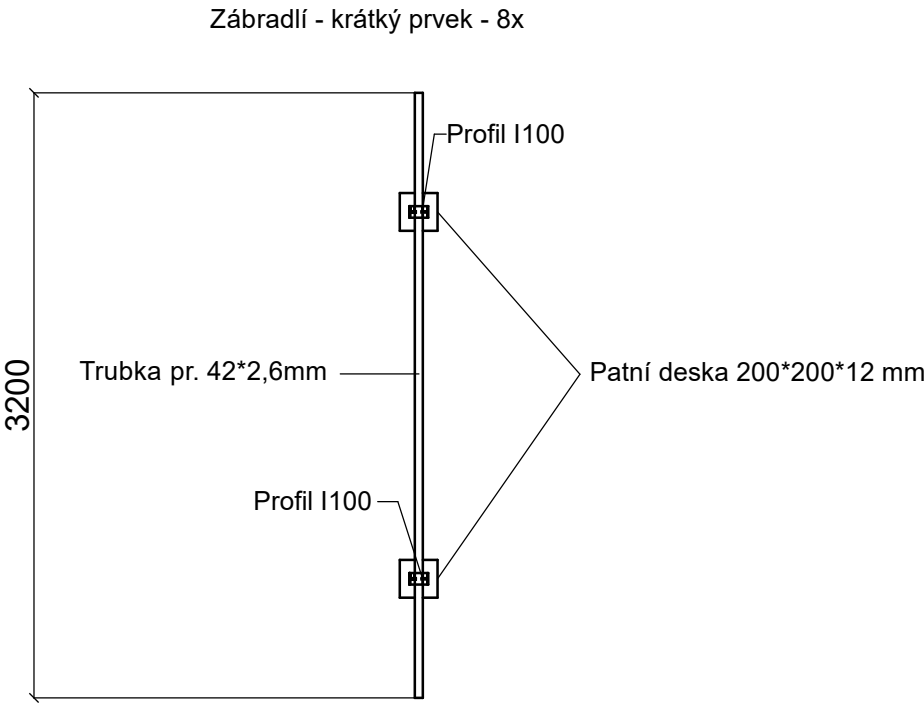
PŮDORYS M 1:40
