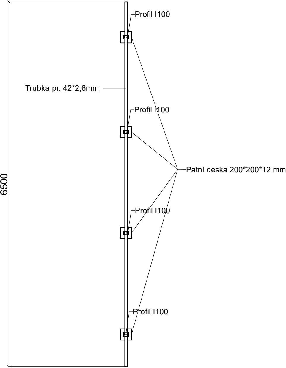
Zábradlí - dlouhý prvek - 3x
