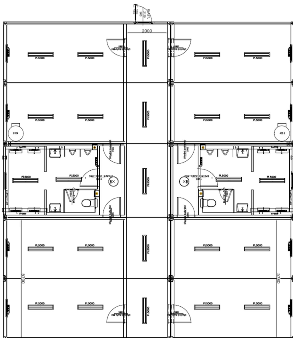
Obr: Příklad vzorového dispozičního řešení kontejnerových šaten (není závazné)
