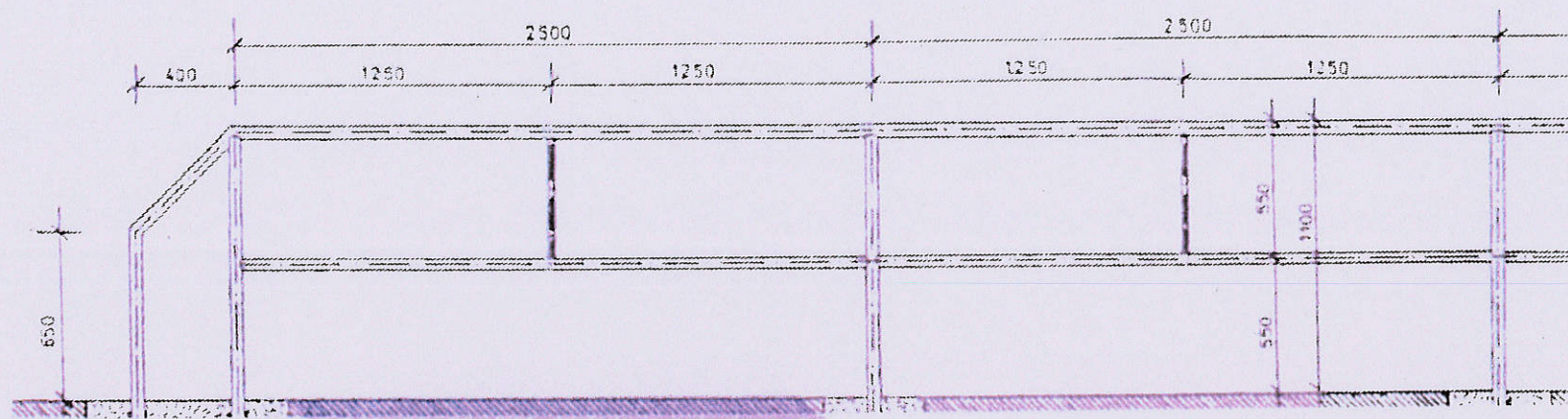
Obrázek 4 – Schéma silničního (dopravně bezpečnostního) zábradlí s výplňovým prutem bez vodící funkce pro nevidomé a slabozraké
